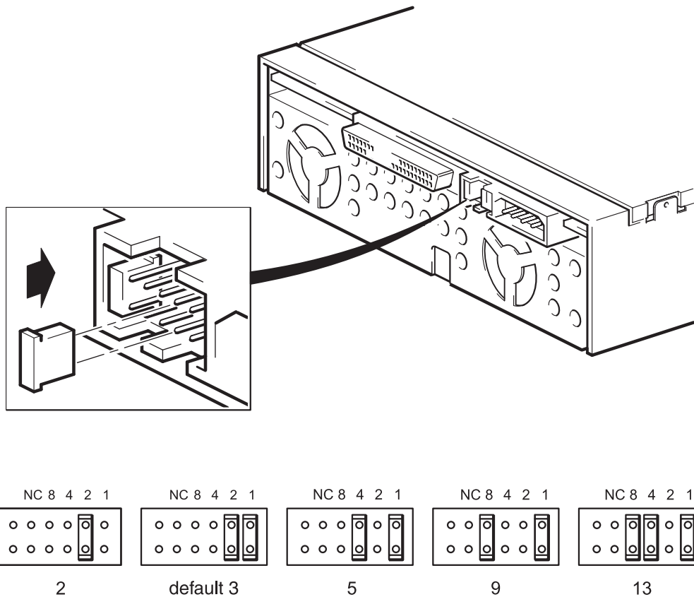
图 3 检查 SCSI ID
